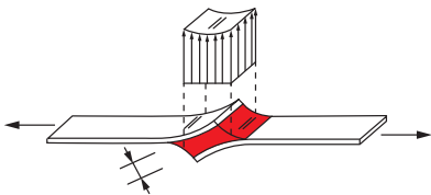
Abb. 1: Größerer Spalt
